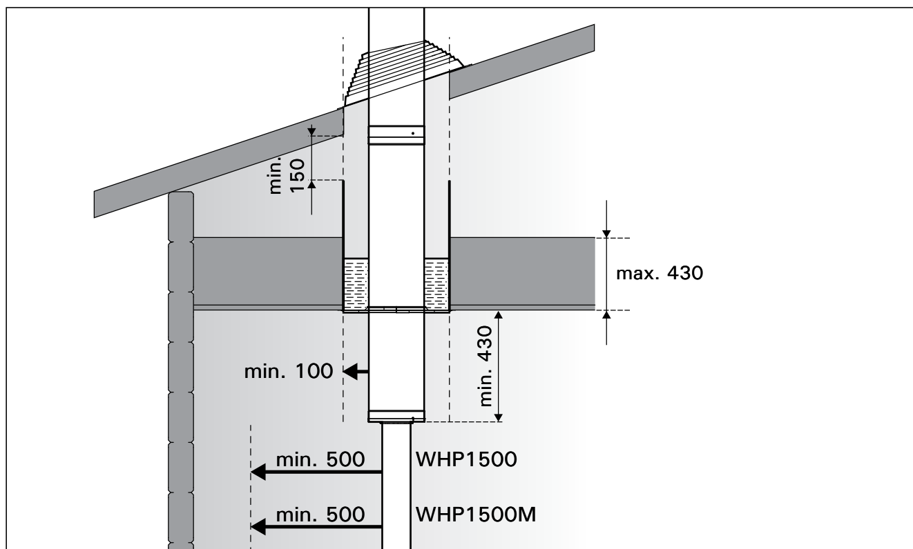
Kuva 2. Suojatäisyydet (mitat millimetreinä) Bild 2. Säkerhetsavstånd (mått i millimeter)
