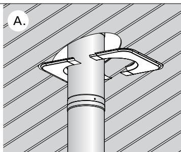
Рисунок 7. Установка проходного фланца
