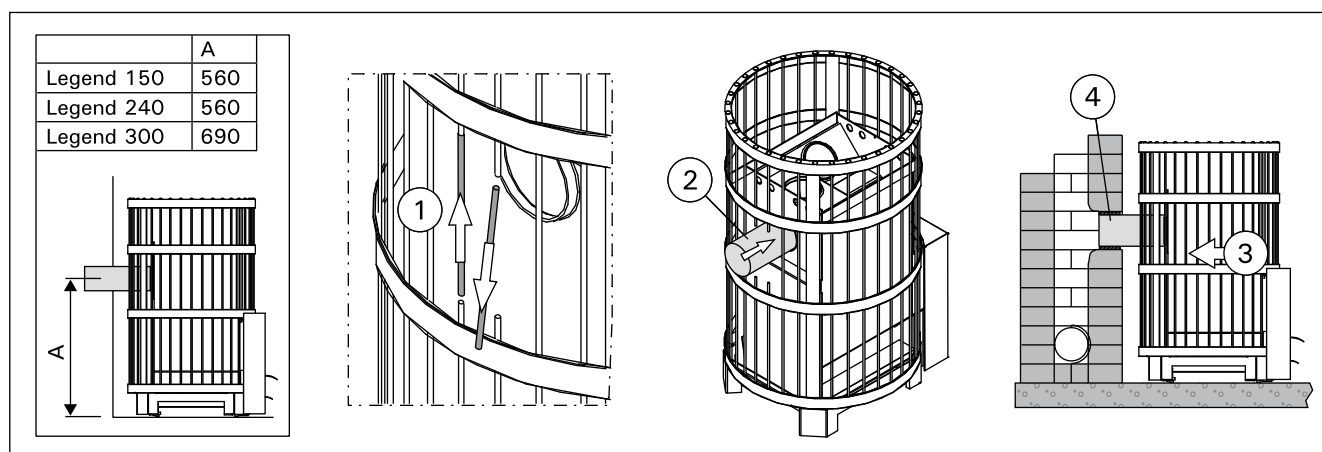
Figure 11. Raccordement du poêle à un conduit maçonné via l'ouverture de raccordement arrière (toutes les dimensions sont fournies en millimètres)
