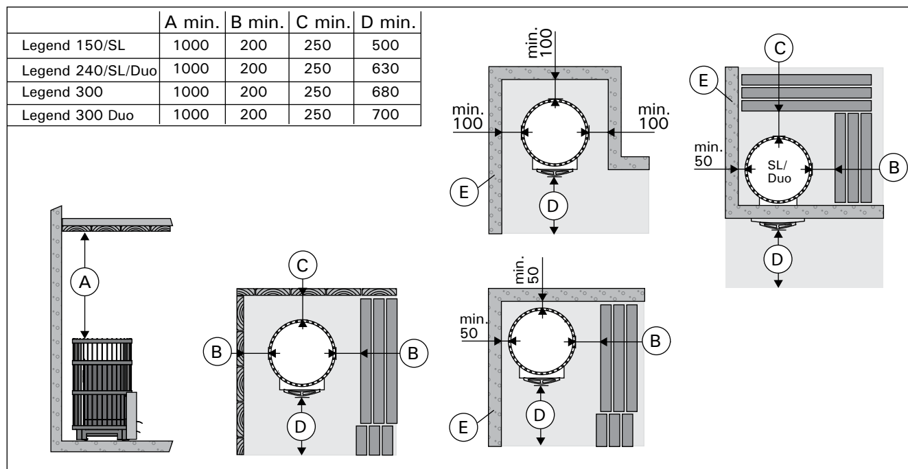
Figuur 9. Veiligheidsafstanden (alle afmetingen in millimeters)
