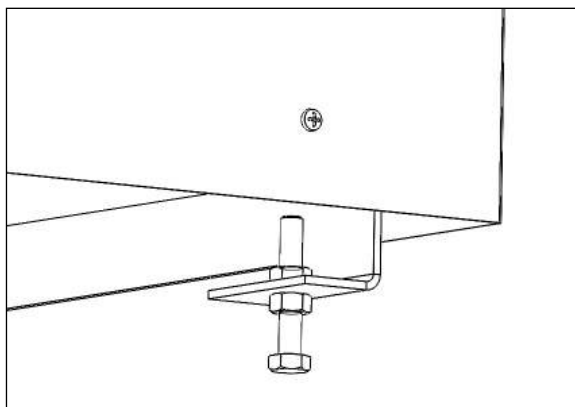
Kuva 2. Säätöjalkojen asennus
